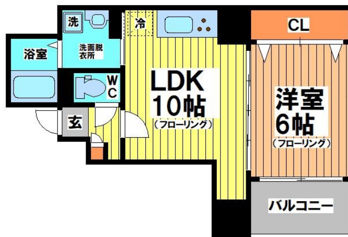
【間取り図】
