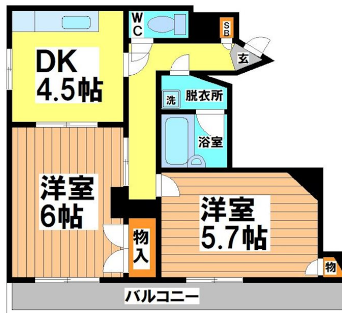
【間取り図】
